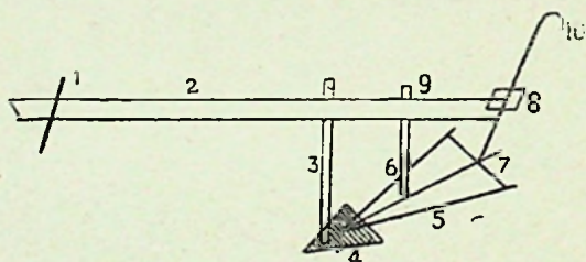
Рало. — Објашњење: 1. клин, 2. војниште, 3. кука, 4. раопник (палечник).. 5. и 6. уши, 7. пречка, 8. клинови, 9. српец (сри) и 10. ручица.
